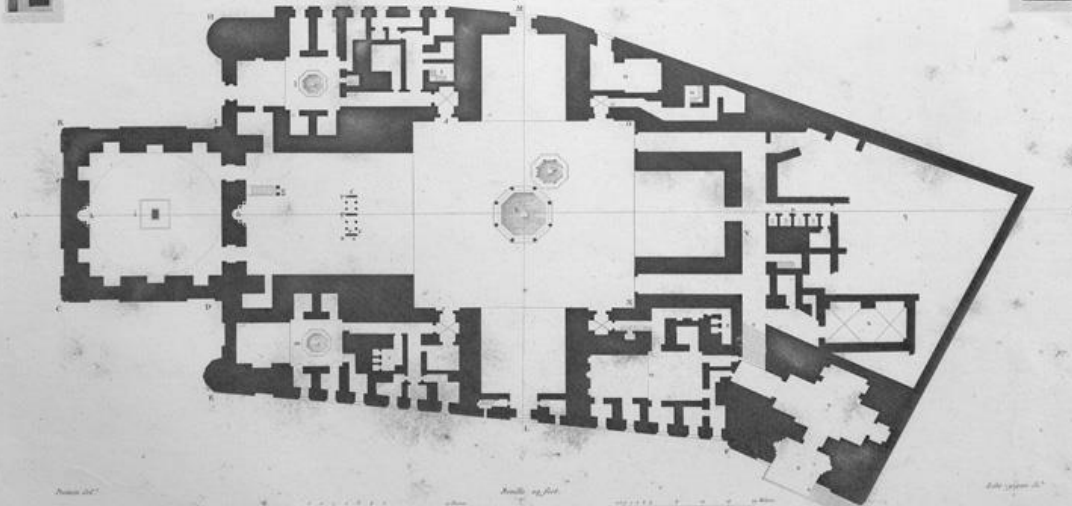
PLAN, ÉLEVATION ET COUPE LONGITUDINALE DE LA MOSQUÉE DE SOULTAN HASAN.
