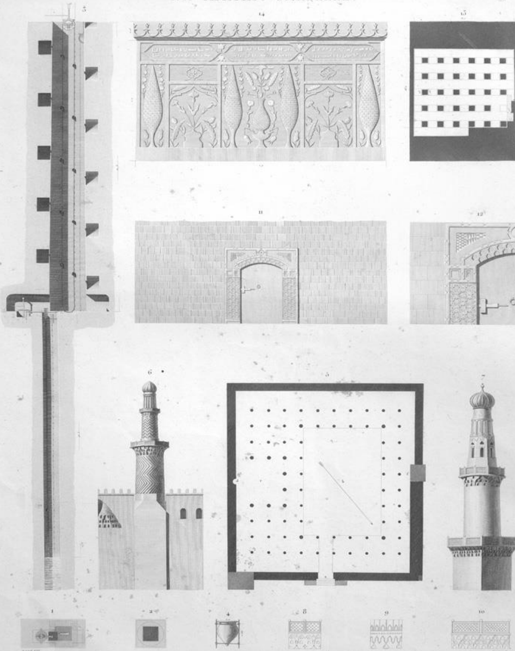
1-4 Puits de Joseph. 5-10 Plan et détails de la Mosquée de Soltan Qalaoun. 11-12 Détails d'une porte. 13 Citerne appelée Sibyl Kikheyd. 14 Tombeau en marbre.
