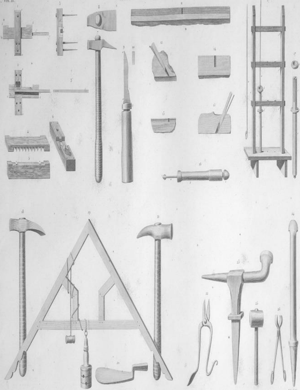
1, 2 SERRENE EGYPTIENNE. 3, 4 AUTRE SERRENE EN BOIS. 5 QADDOCH OU ESSETTE. 6 BEC D'ANE. 7 VEILLERET. 8, 9 DEUX RABOTS. 10 FORET. 11 MACHINE A FORER LES TUYAUX DE PIPE. 12, 13, 14 Outils du MAÇON. 15, 16 Outils du CHAUDRONNIER ET DU FERBLANTIER.
