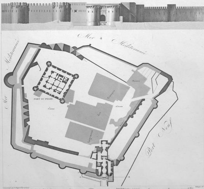
1. 2 VUES DU CHATEAU DU PIARE ET DU ROCHER DU DIAMANT. 4. 5 PLAN ET ÉLEVATION DU CHATEAU DU PIARE.
