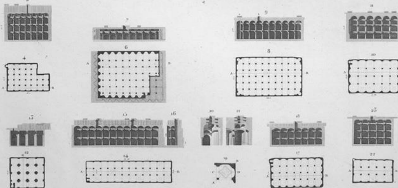
1. 2. 3. PLAN, ÉLEVATION ET COUPE D'UNE ANCIENNE ÉGLISE DITE MOSQUÉE DES MILLE COLONNES OU DES SEPTANTE. 4. 25 PLANS, COUPES ET DÉTAILS DE HUIT DES PRINCIPALES CITERNES DE L'ANCIENNE VILLE.
