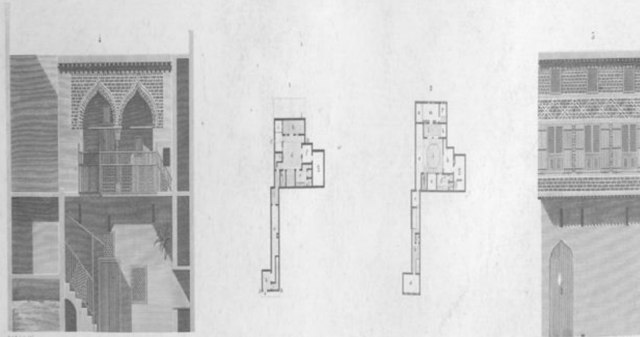
PLANS, COUPES, ÉLEVATIONS ET DÉTAILS DE MENUISERIE D'UNE MAISON TURQUE.
