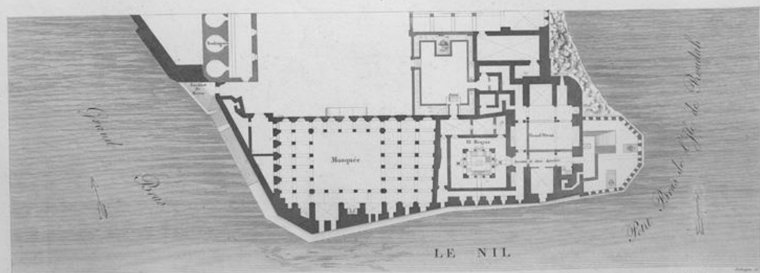
PLAN GÉNÉRAL DU MEQYAS OU NILOMÈTRE. PLAN DU Puits. COUPE DU NILOMÈTRE. DÉTAILS DE LA COLONNE.
