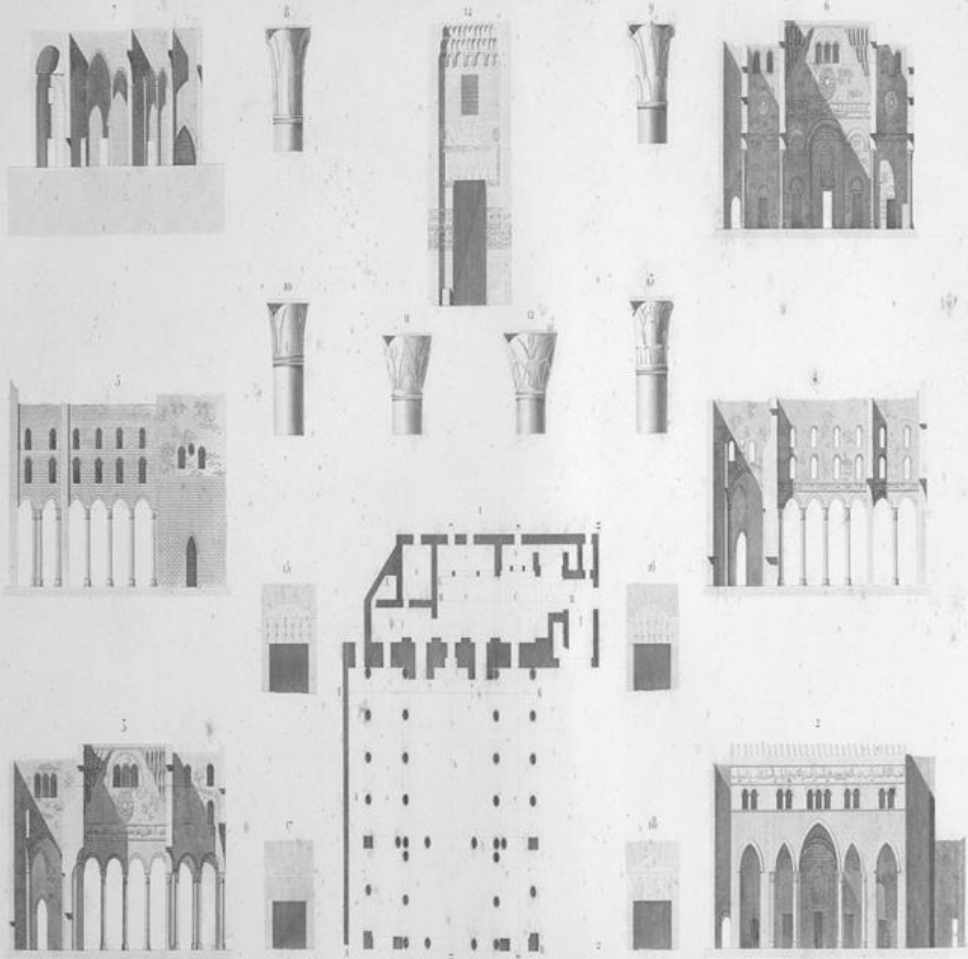
1. 3 PLAN, ELEVATIONS, COUPES ET DÉTAILS DE CHAPITRAUX DE DIVAN DE JOSEPH. 11. 10 DÉTAILS DE PORTES.
