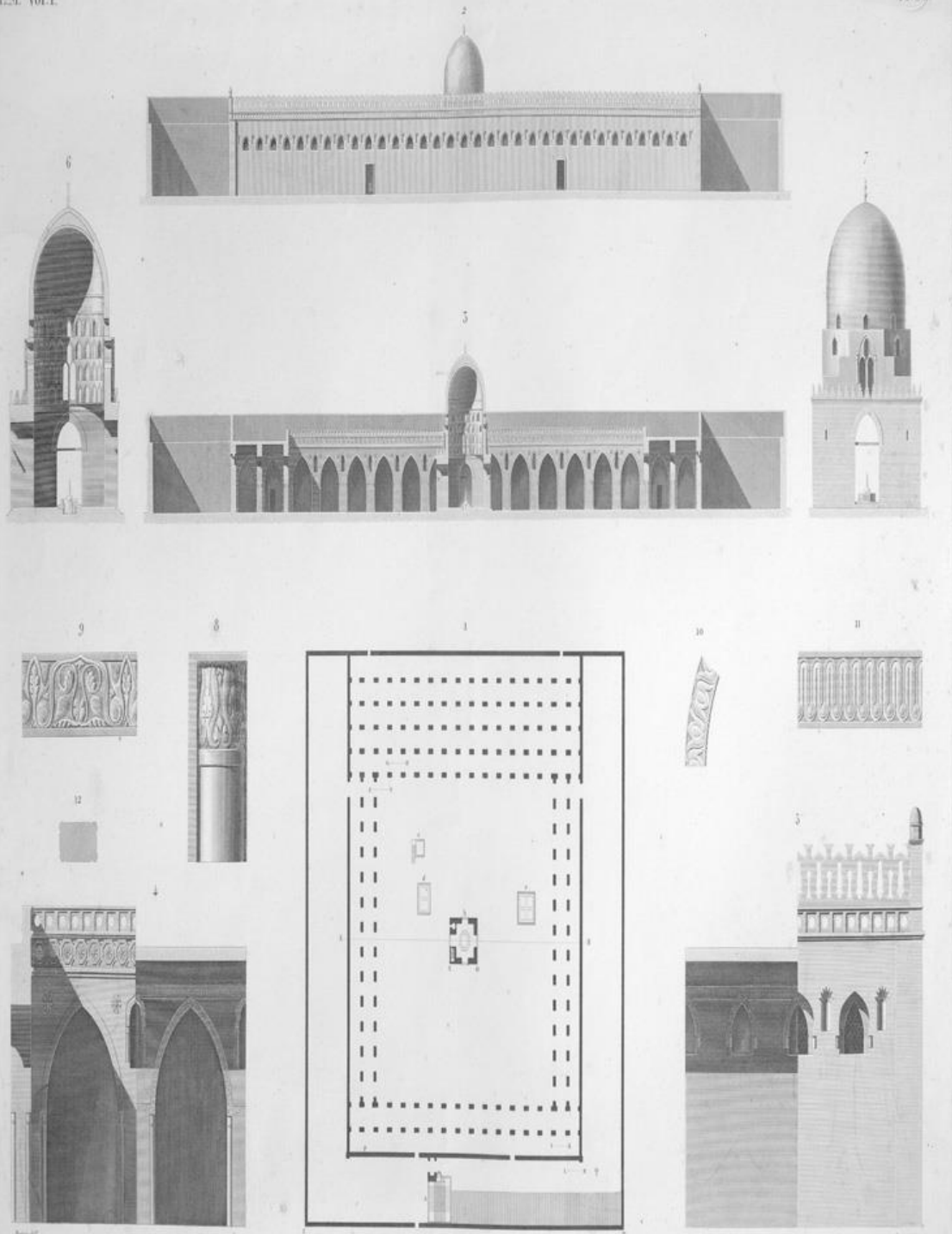
PLAN, ELEVATION, COUPES ET DÉTAILS D'ORNEMENT DE LA MOSQUÉE DE TOULOÛX.
