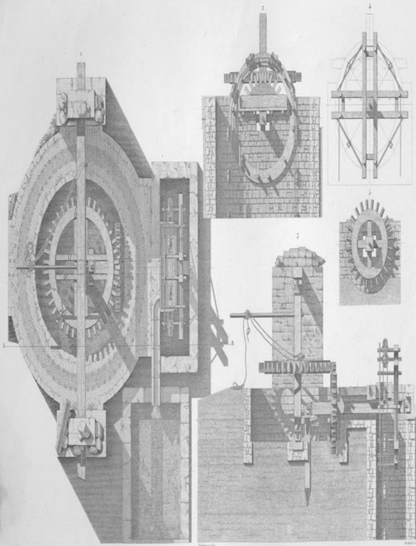
PLAN, COUPE ET DÉTAILS DE LA ROUE A POTS OU MACHINE A ARROSER.
