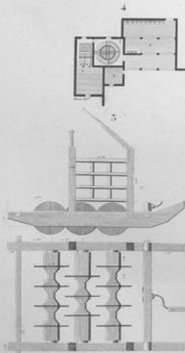
1 CHARRUE. 2 MACHINE A BATTRE LES GRAINS. 3 - MACHINE A BLANCHIR LE RIZ. 4, 5 MOULIN A FARINE.
