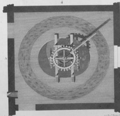
VUE. PLANS ET COUPES DU MOULIN A SUCRE.
