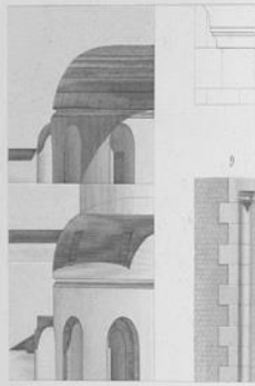
1. VUE DE TROIS COLONNES EN GRANT, SITIÉES AU SUD DE L'ANCIENNE BASILIQUE VULGAIREMENT NOMMÉE MOSQUÉE DE S. ATHANASE. 2. 9 VUE INTÉRIÈRE, PLANS, COUPES ET DÉTAILS D'UNE TOUR ANTIQUE, PLACÉE AU NORD DES DEUX OBÉLISQUES, ET CONNUE SOUS LE NOM DE TOUR DES ROMAINS.
