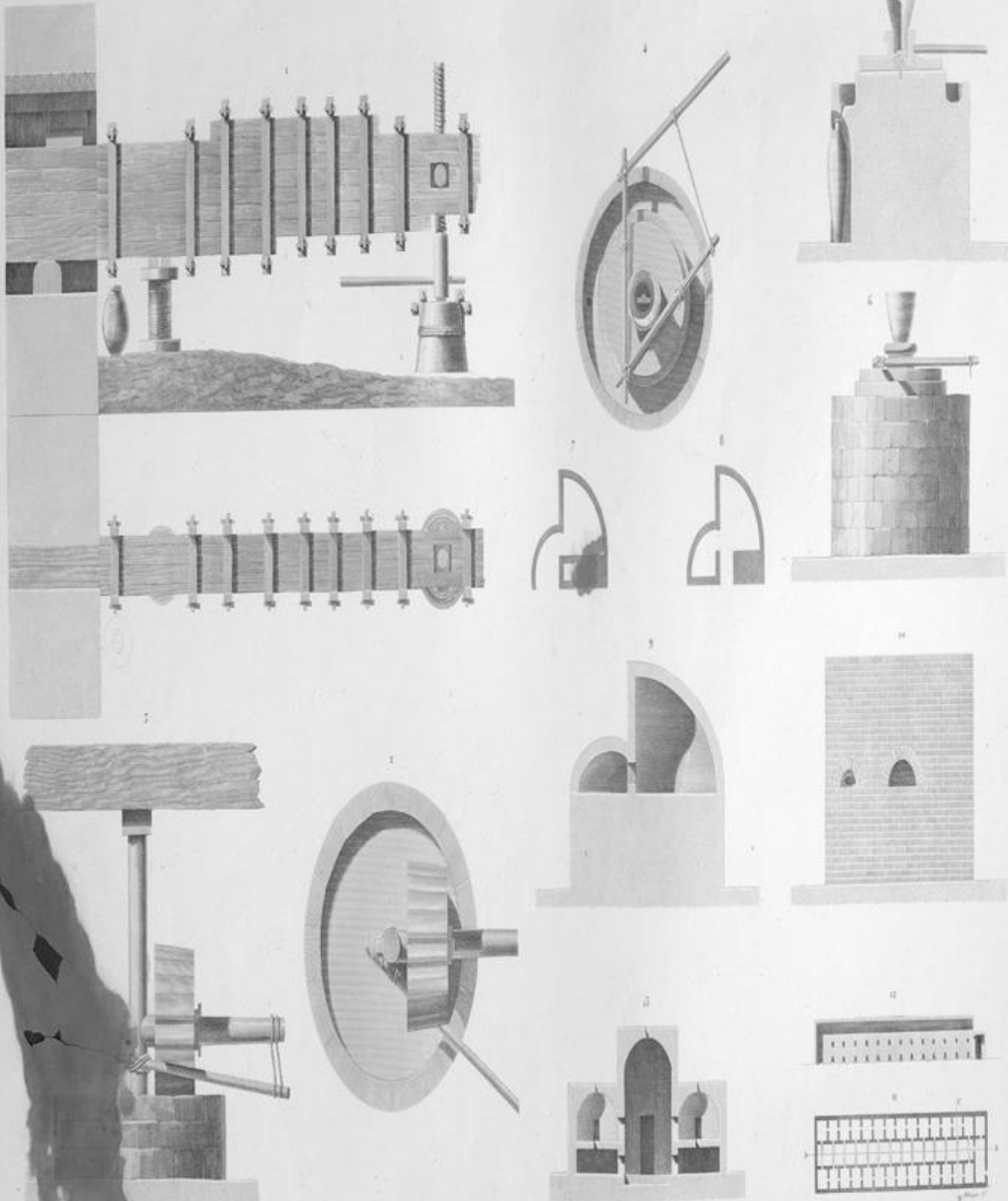
1. PRESOIR A HUILE DE LIN. 2. MOULIN A HUILE DE LIN. 3. MOULIN A HUILE DE SESAME. 4. 5. FOURNEAU A TORREFIER LA GRAINE DE SESAME. 6. 7. FOUR A POULETS DE LOUQUEUR.
