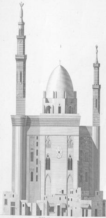
1. 2. ÉLEVATION ET COUPE TRANSVERSALE DE LA MOSQUÉE DE SOULTAN HASAN. 3. DÉTAIL DE LA PORTE D'ENTRÉE.
