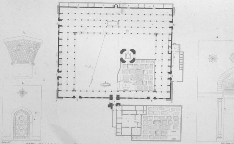
PLAN, ÉLEVATION, COUPE ET DÉTAILS D'UNE ANCIENNE BASILIQUE, VULGAIREMENT NOMMÉE MOSQUÉE DE S T . ATHANASE.
