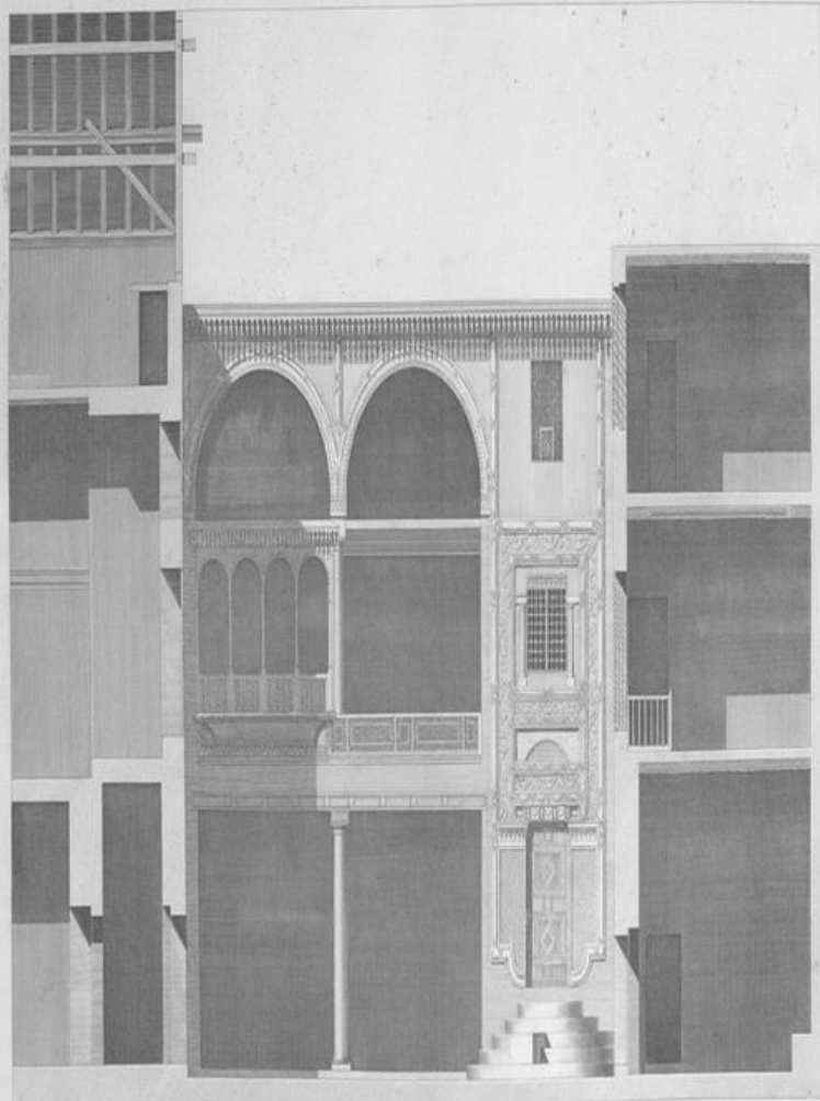
COUPE DE LA MAISON D'YBRAHIM KIKHEVD EL SENNARY.
