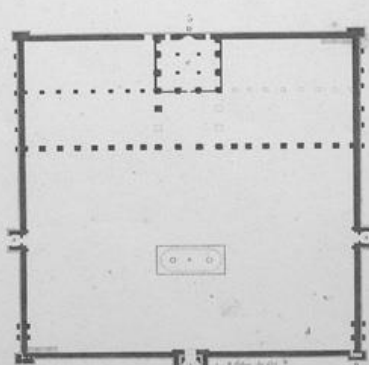
1, 2, 3, 4 PLANS DE PLUSIEURS GRANDES MOSQUÉES. 5, 6-8 PLAN, ÉLEVATIONS ET COUPE DE LA MOSQUÉE APPELÉE GÂM' EL DÂHER. 9 PONTS SITUÉS SUR LE CANAL DU KAIRE.
