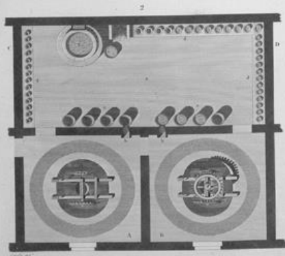
VUE. PLANS ET COUPES DU MOULIN A SUCRE.
